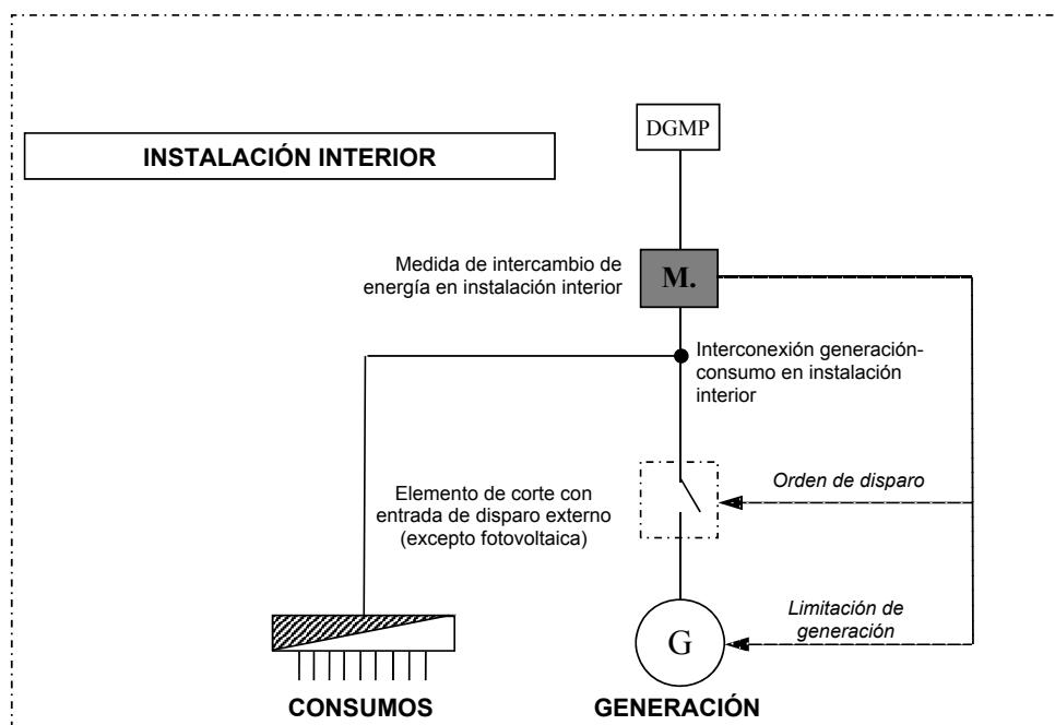
Figura 1: Esquema con equipo de medida de intercambio de energía con la red en instalaciones conectadas a redes de baja tensión
